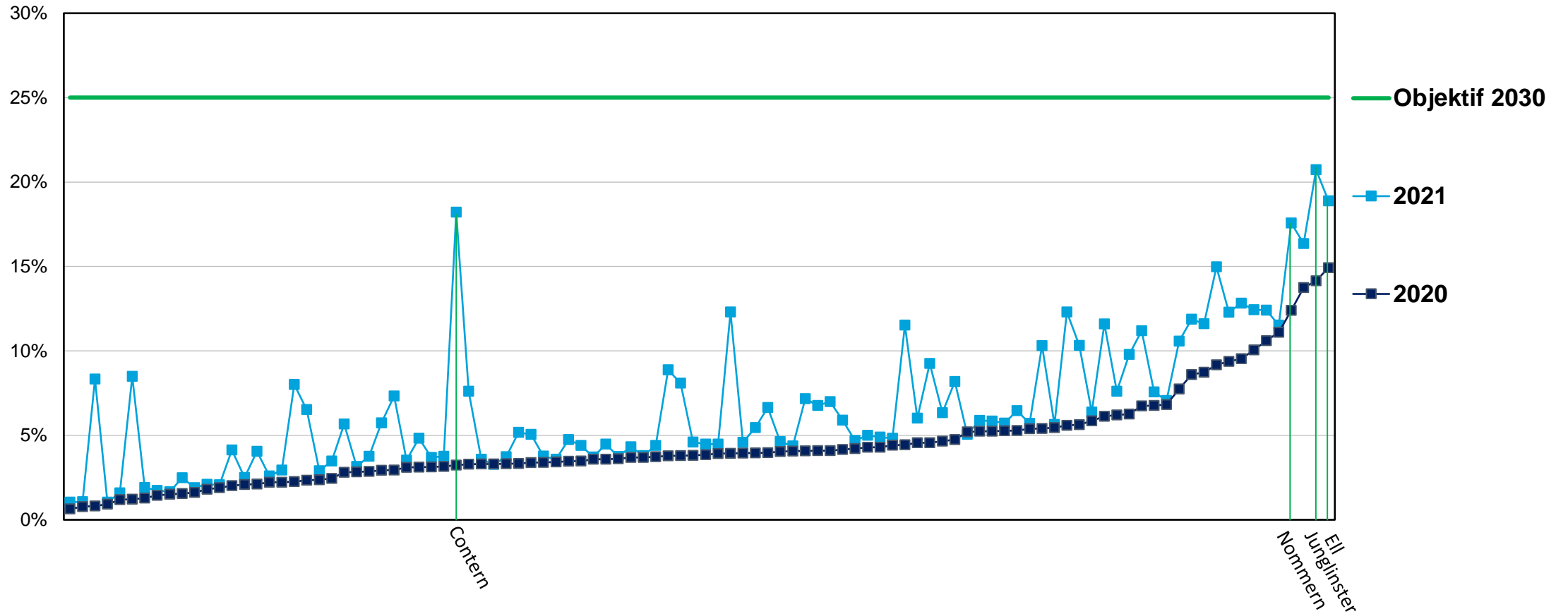
KPI 3.2.1 : Puissance photovoltaïque installée / potentiel
